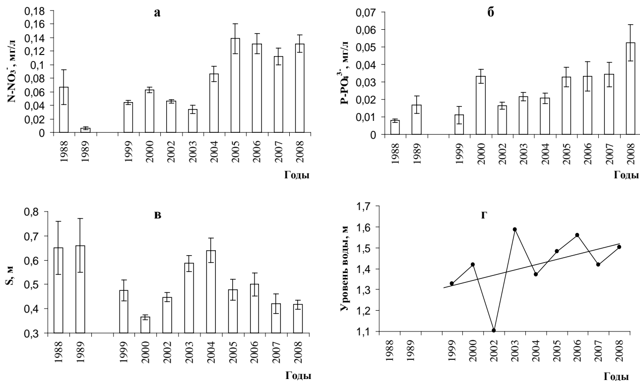
Рис. 2. Многолетние изменения средних за безледный период (V-X): а – концентраций нитратного азота; б – концентраций минерального фосфора; в – значений прозрачности воды; г – значений уровня воды.
